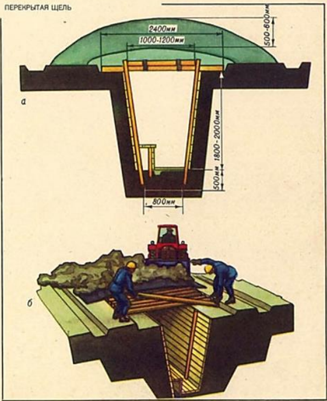
а) схема щели; б) сооружение перекрытой щели с одеждой кругостей
